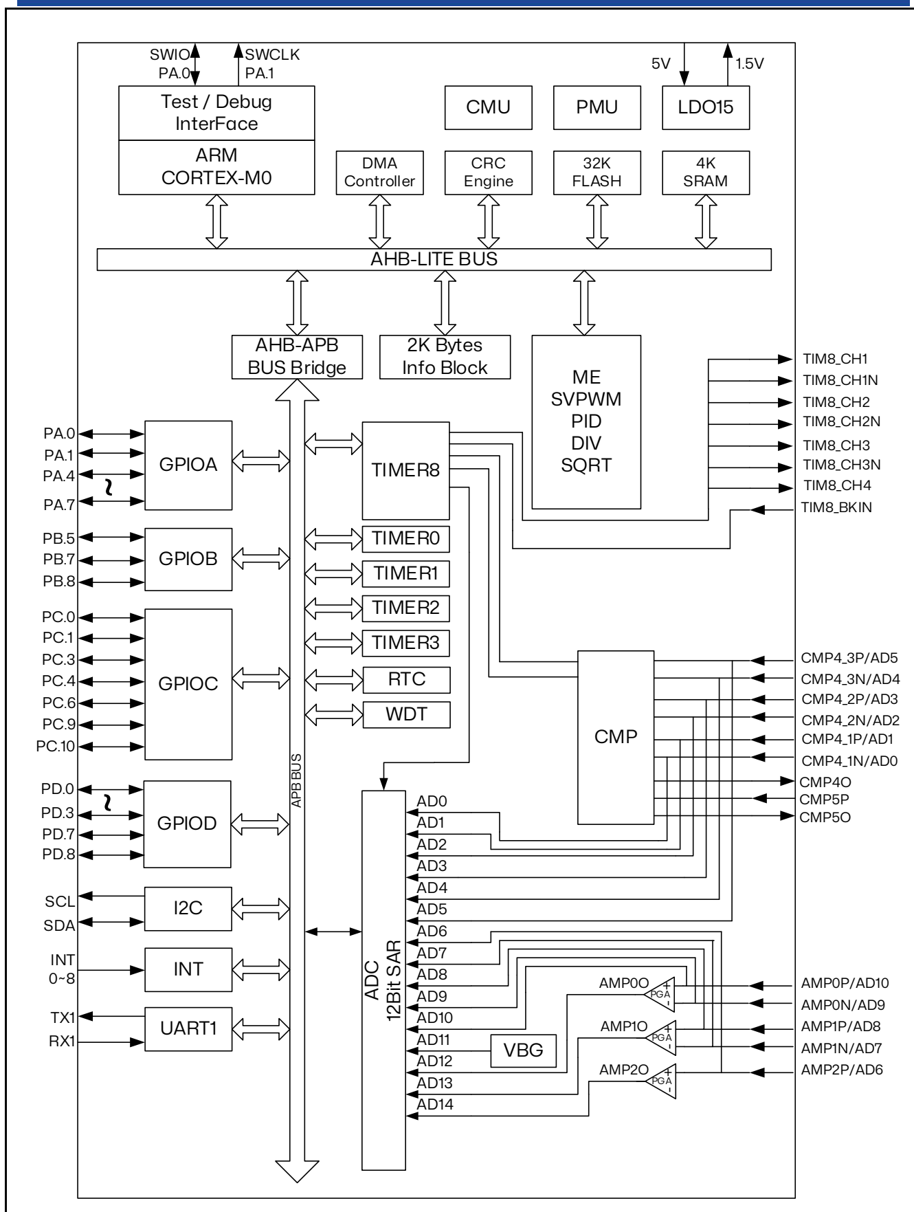
图 2.1 RX32S11 架构图
