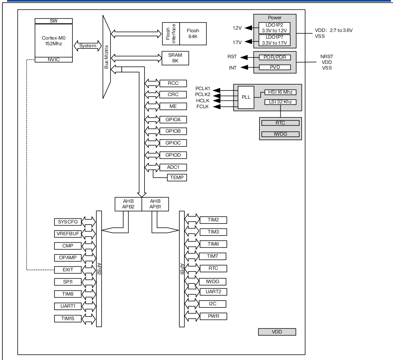
图 2.1 RX32S610 架构图
