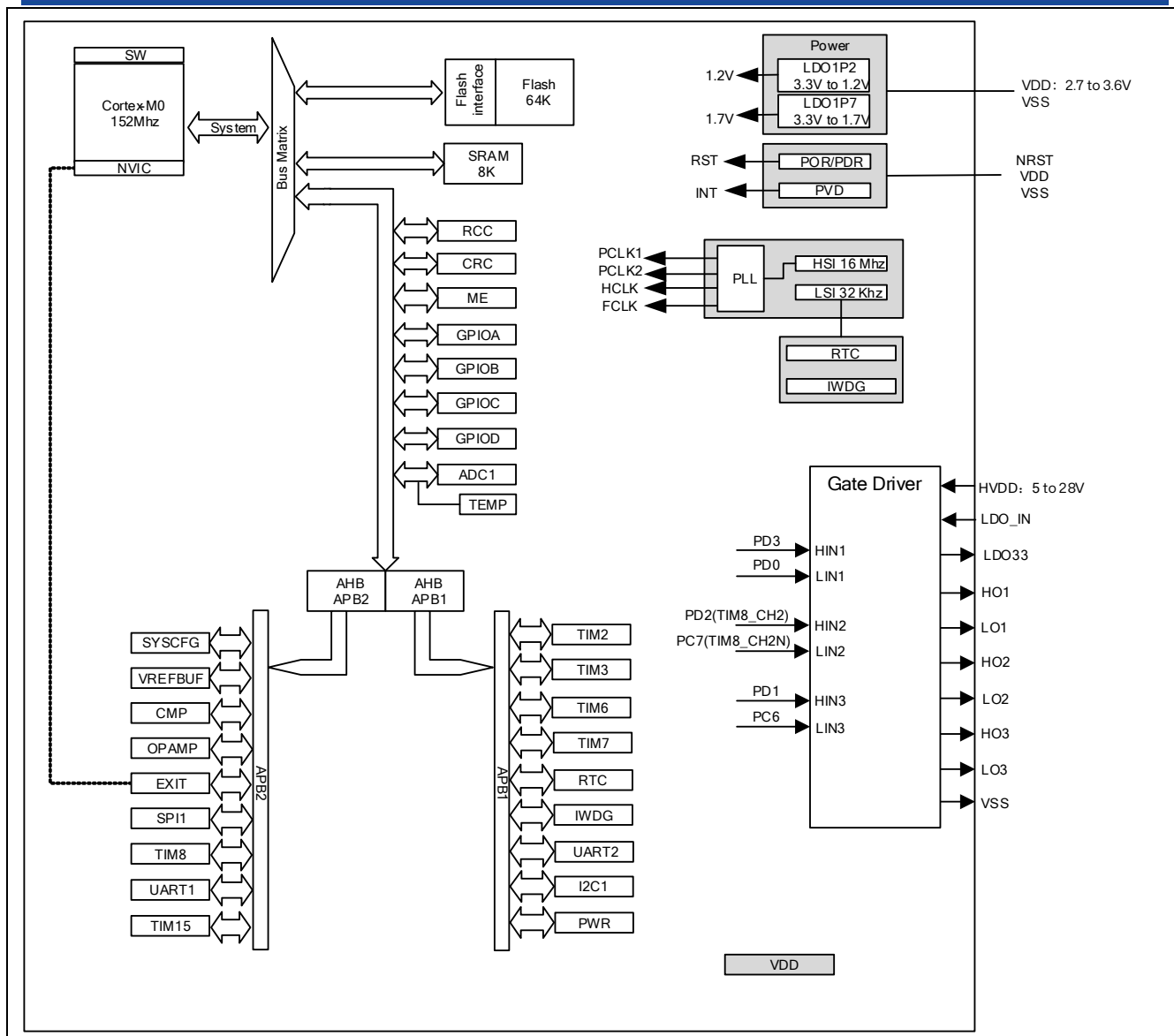
图 2.1 RX32S632 架构图
