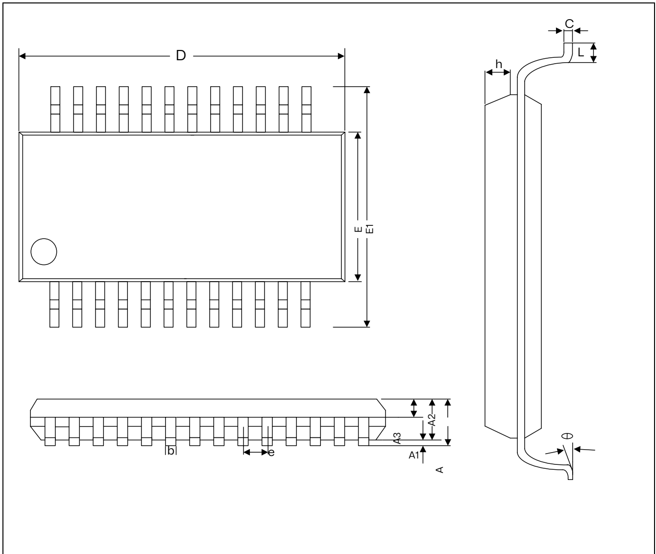
图 6.1 轮廓图
