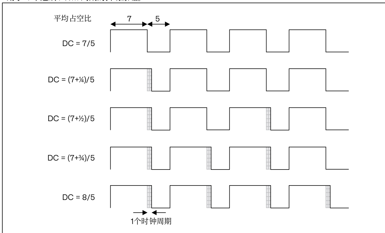
图 15.34 抖动原理
