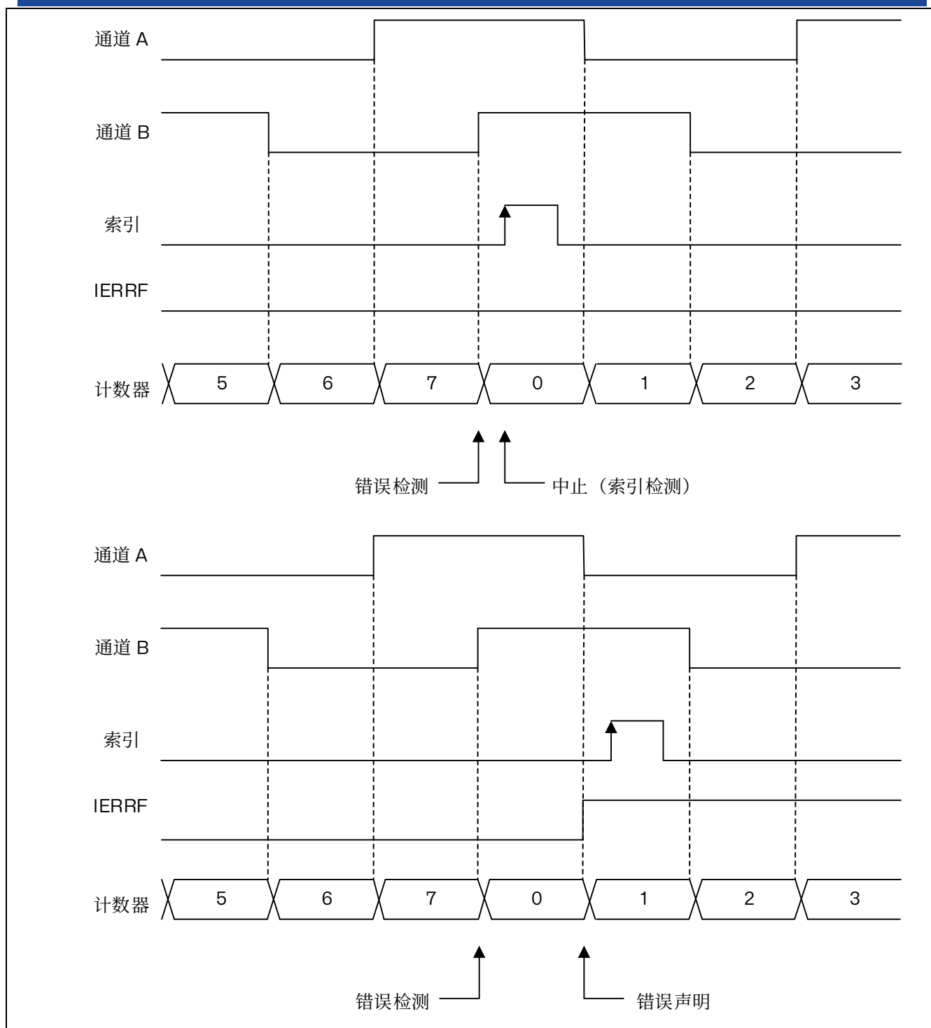
图 15.72 递增计数编码器错误检测
