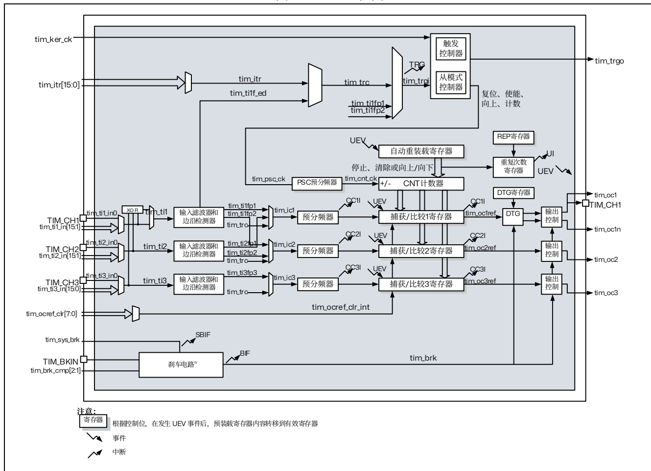
图 16.1 TIM15 框图
