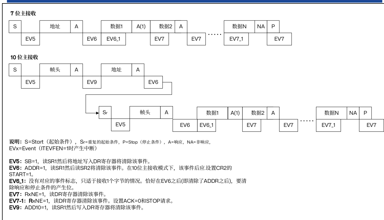
图 24.6 主接收器传送序列图
