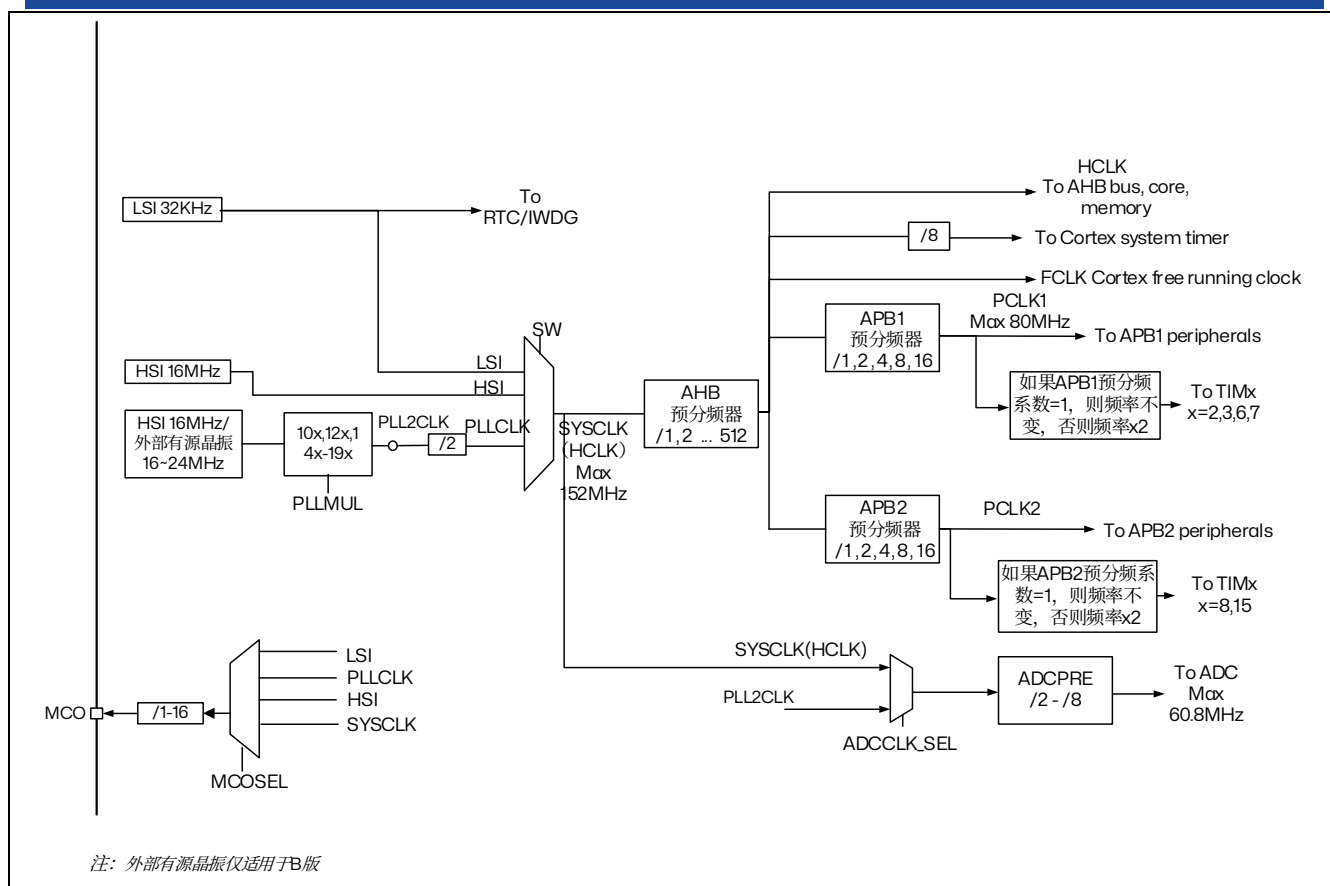
图 7.2 时钟树
