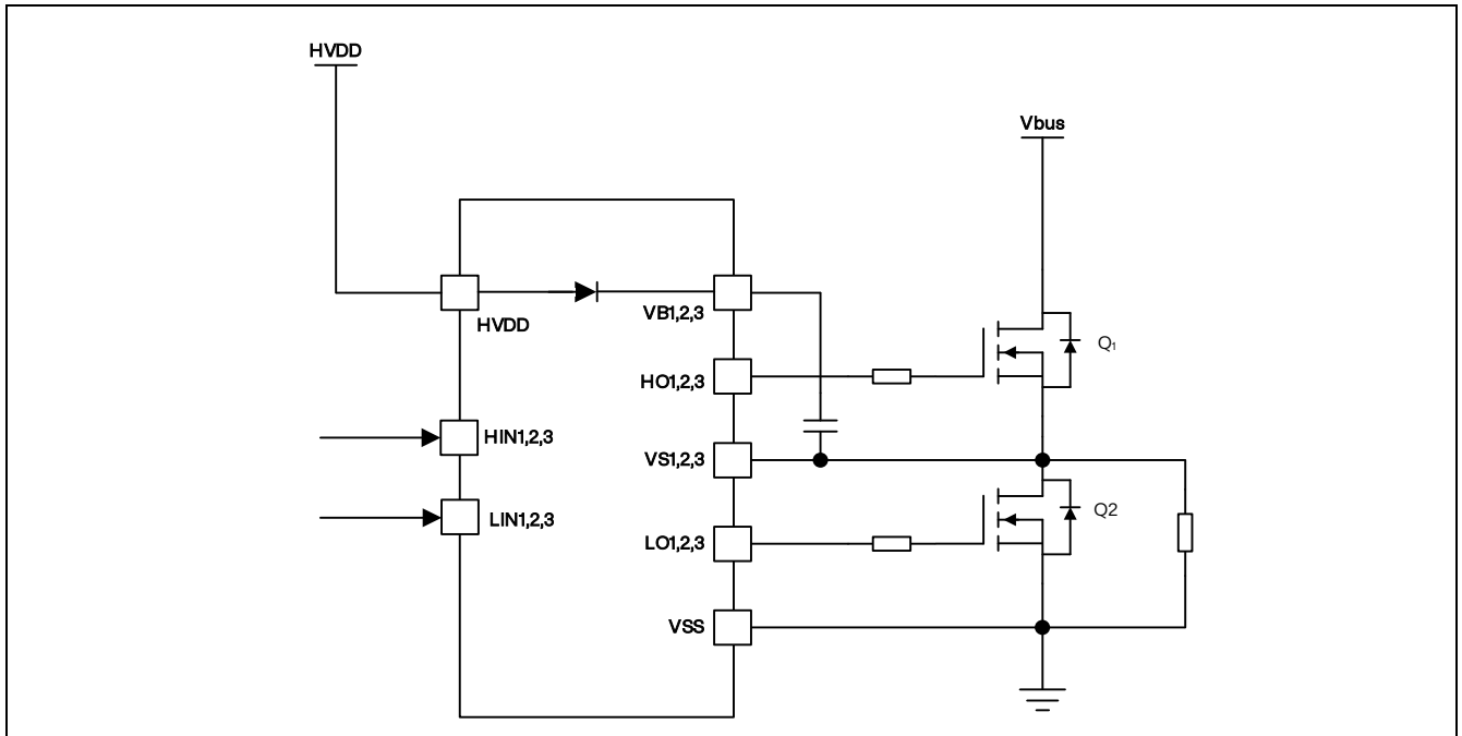
图 26.3 应用电路
