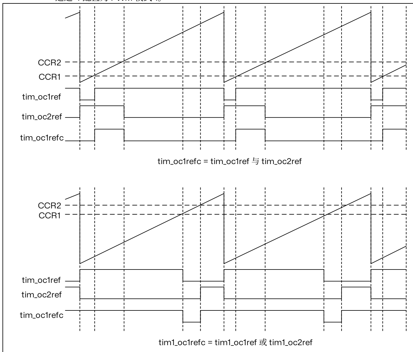
图 14.41 通道 1 和通道 3 的组合 PWM 模式
