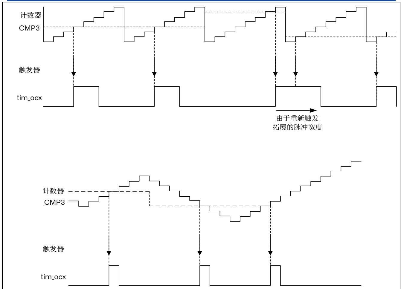
图 14.57 在比较事件上的脉冲生成，适用于边沿对齐模式
