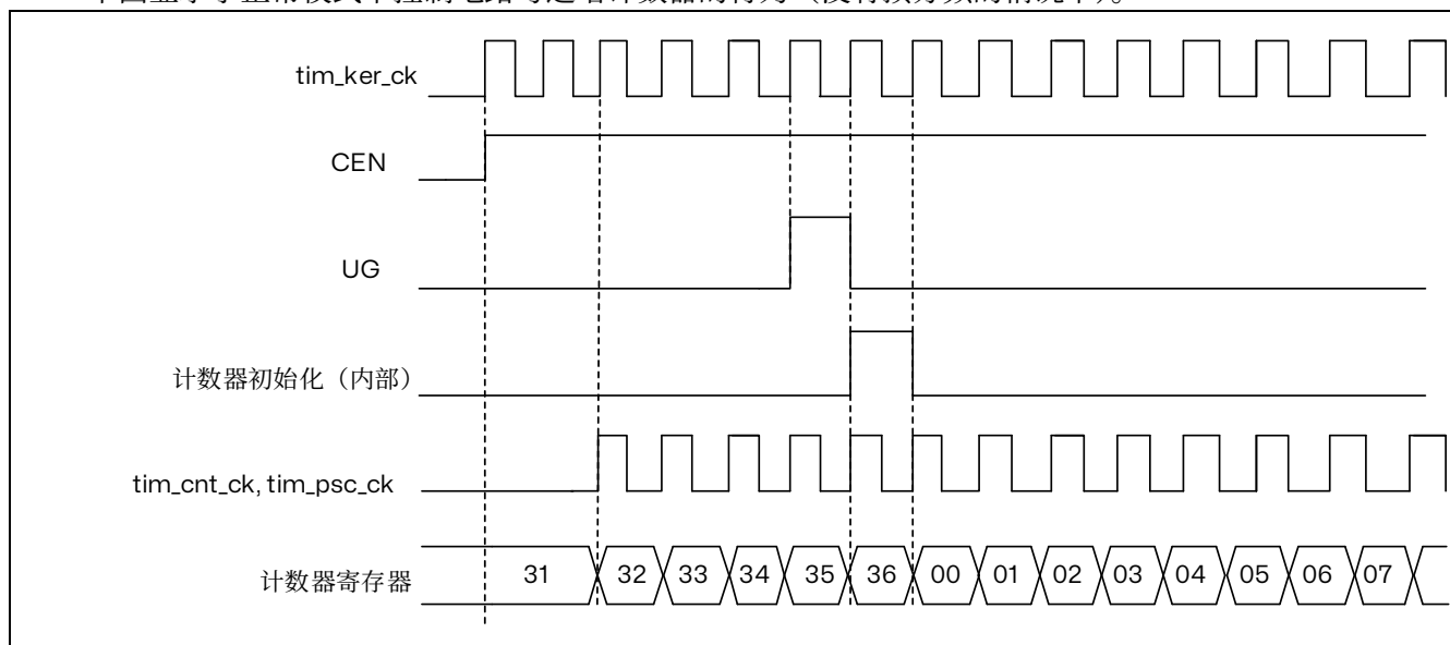
图 16.11 一般模式下的控制电路，内部时钟分频因子为 1
