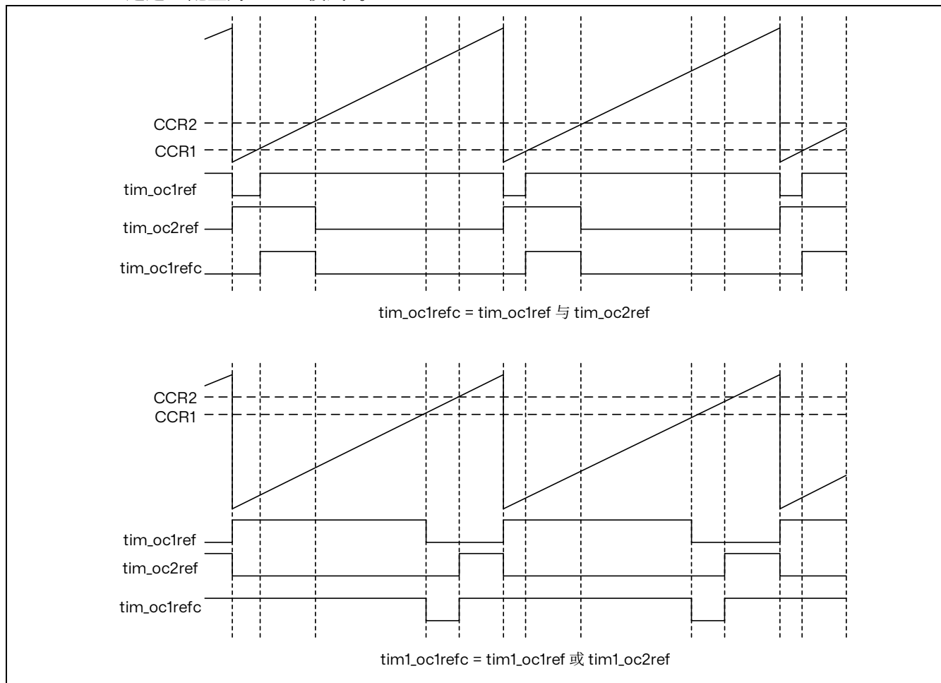
图 15.43 通道 1 和通道 3 的组合 PWM 模式
