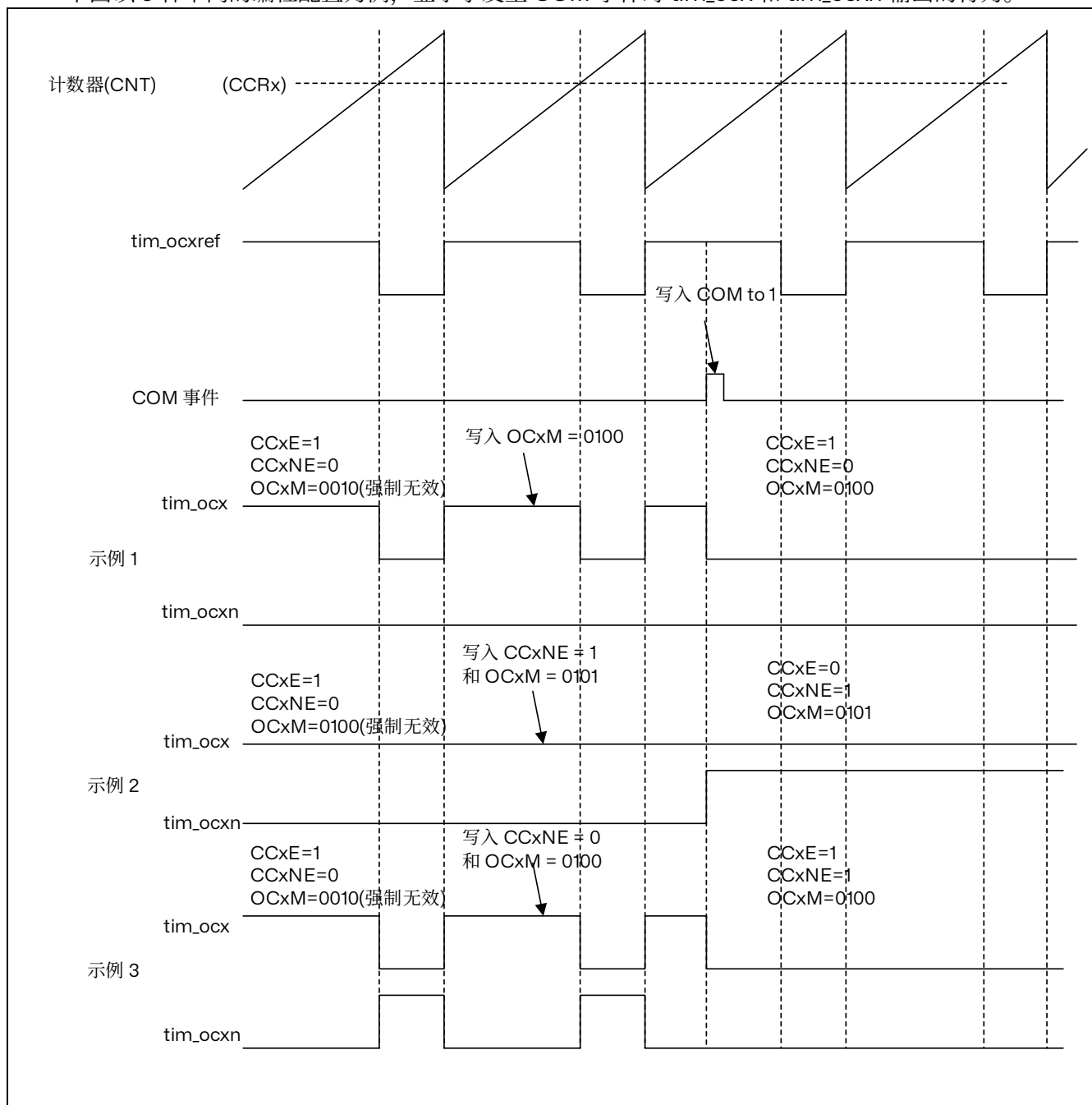
图 14.53 COM 事件生成 6 步 PWM 的示例 (OSSR=1)
