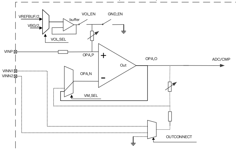
OPAMP1/OPAMP2: FOLLOW MODE (P-IO_N-OUT)
