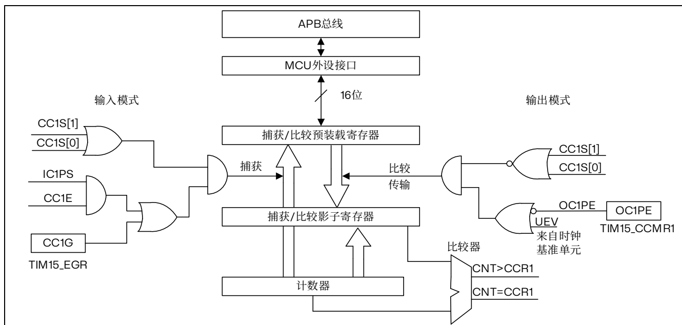
图 16.15 捕获/比较通道1的主电路
