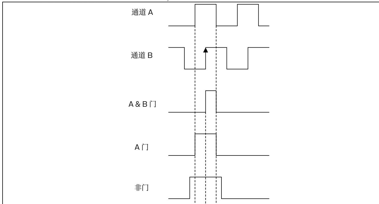
图 15.57 索引门控选项
