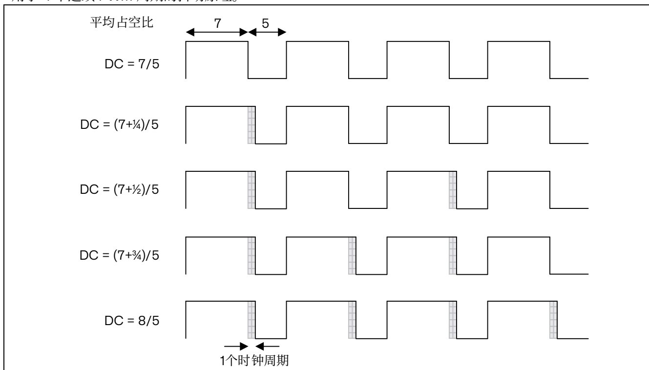
图 15.33 抖动原理
