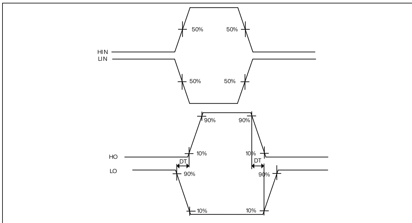
图 26.2 死区时间波形图
