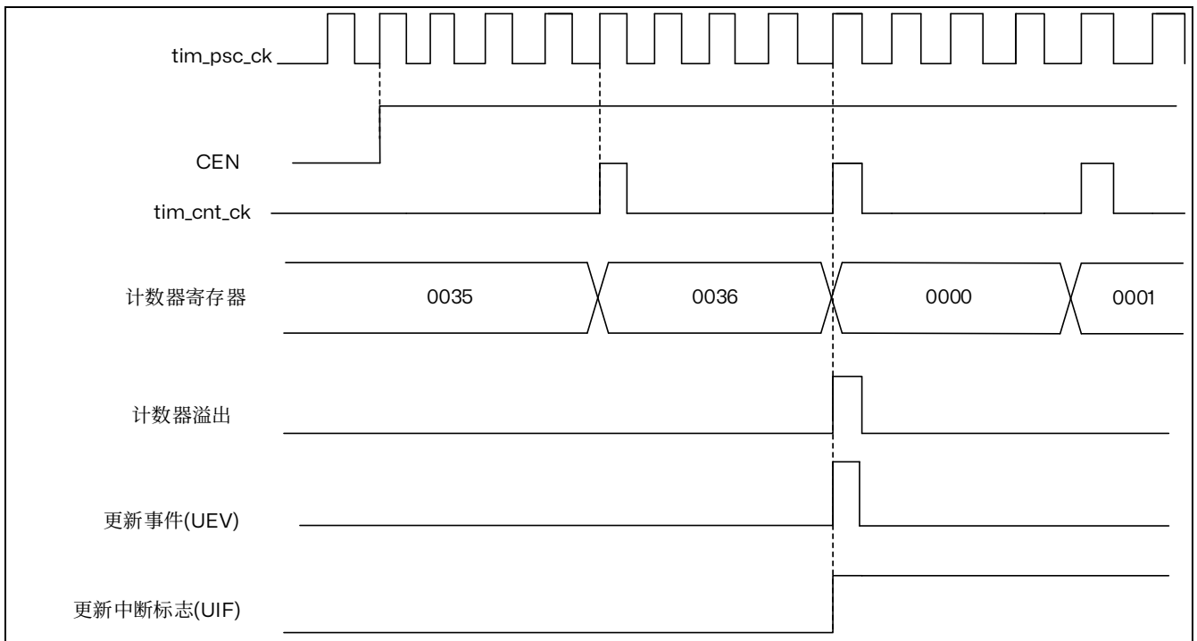
图 14.6 计数器时序图，内部时钟分频因子为 4
