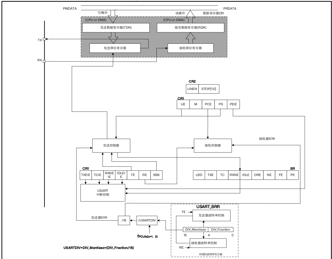
图 25.1 UART 框图
