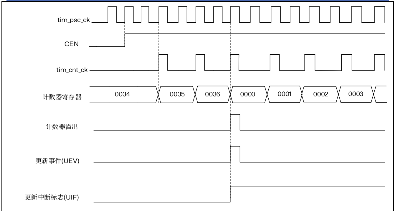
图 14.5 计数器时序图，内部时钟分频因子为 2
