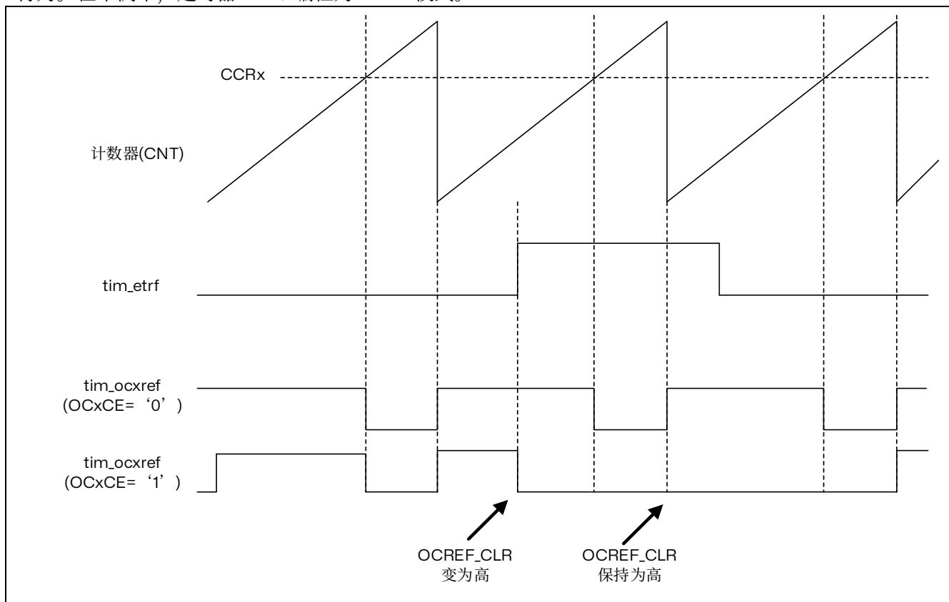
图 14.52 清除 TIM8 的 tim_ocref
