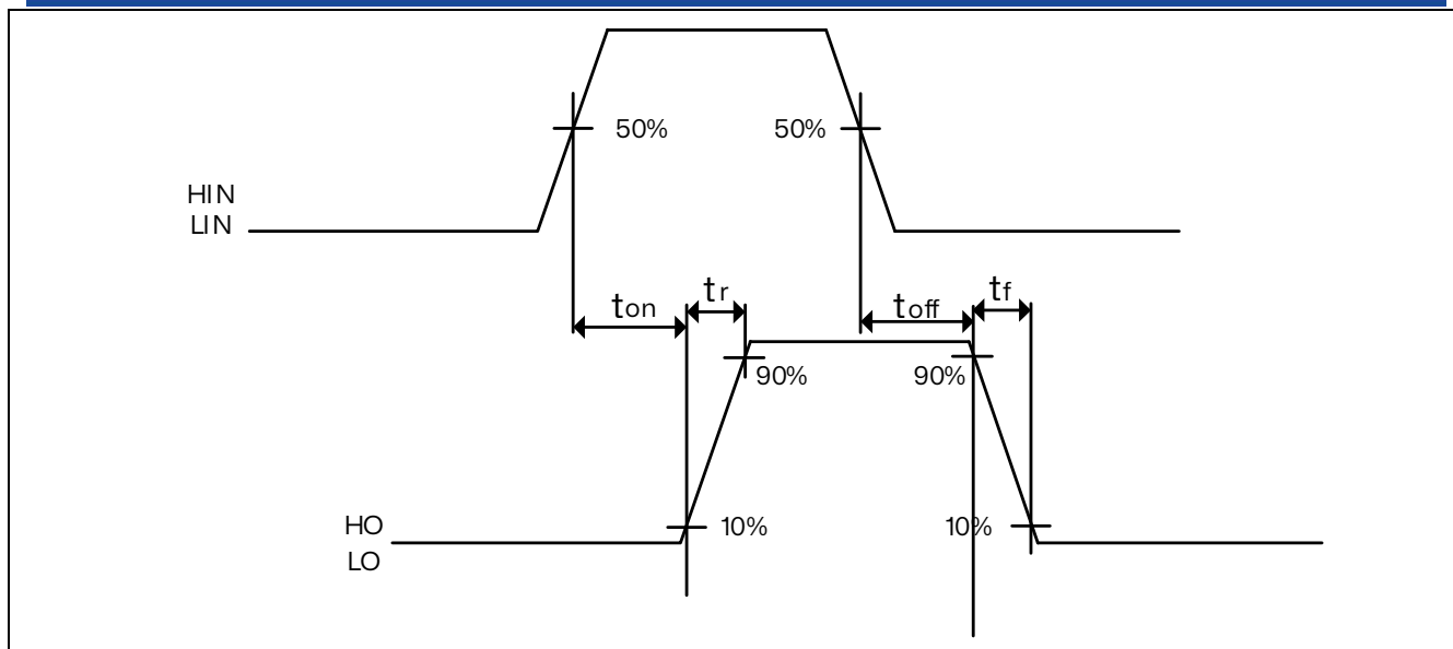
图 26.1 时间切换波形图
