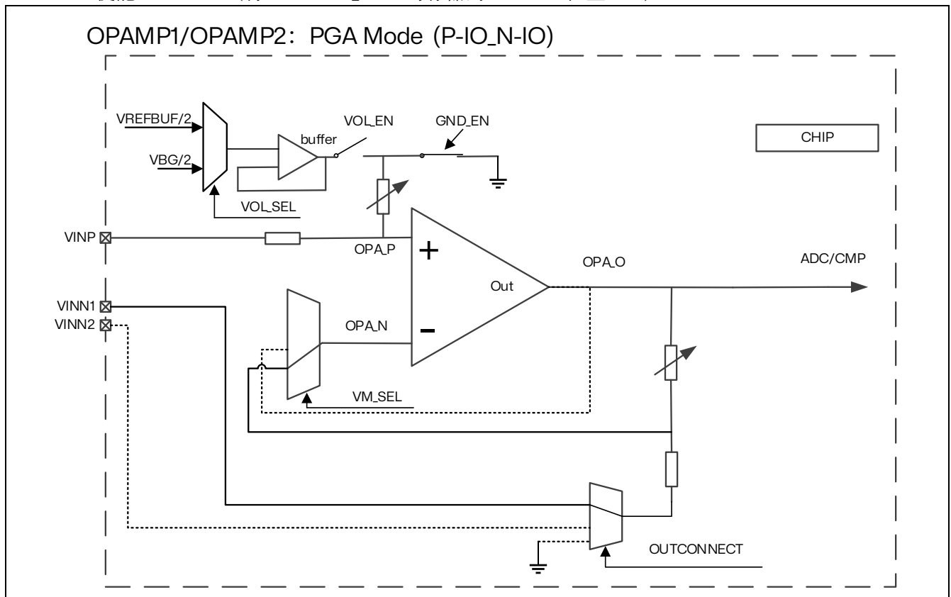
图 18.4 OPAMP1/OPAMP2 PGA 模式 (P-IO, N-IO)
