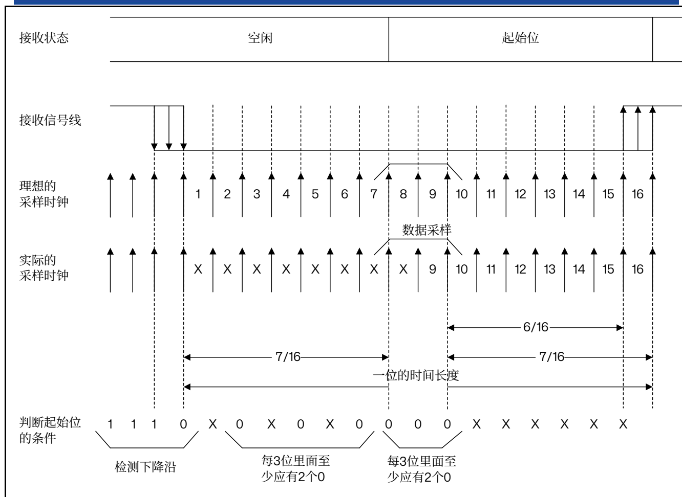
图 25.5 起始位侦测
