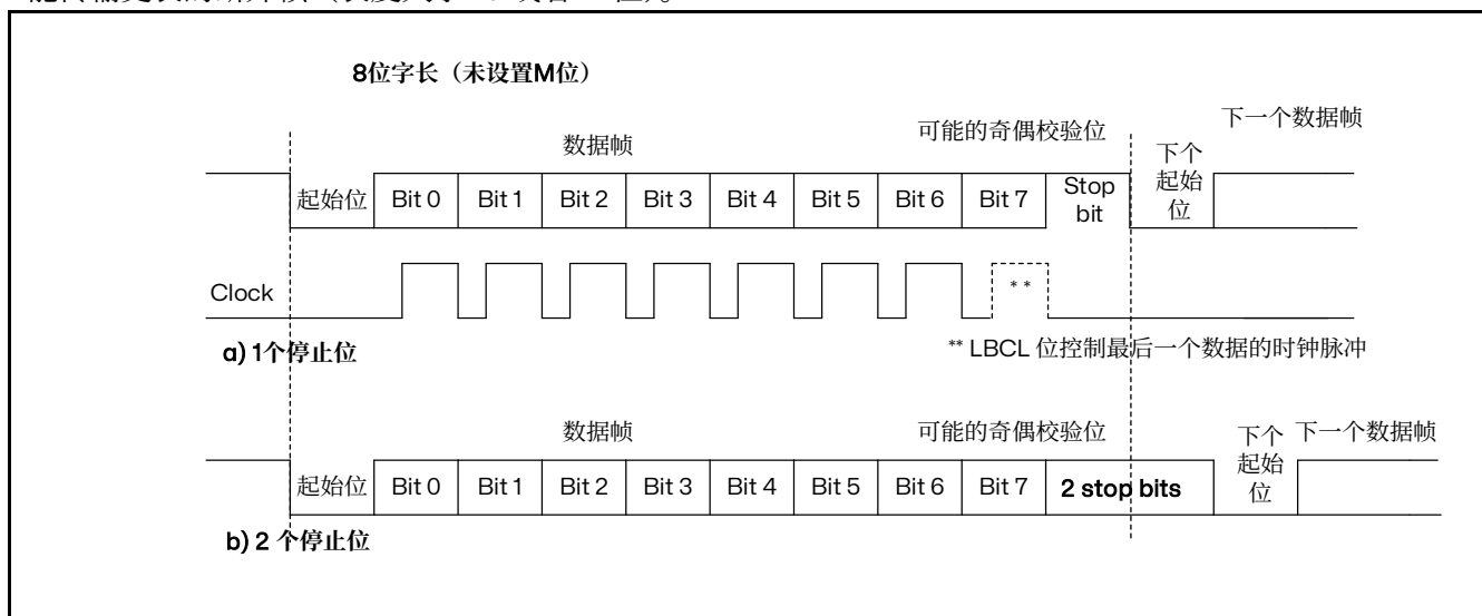
图 25.3 配置停止位
