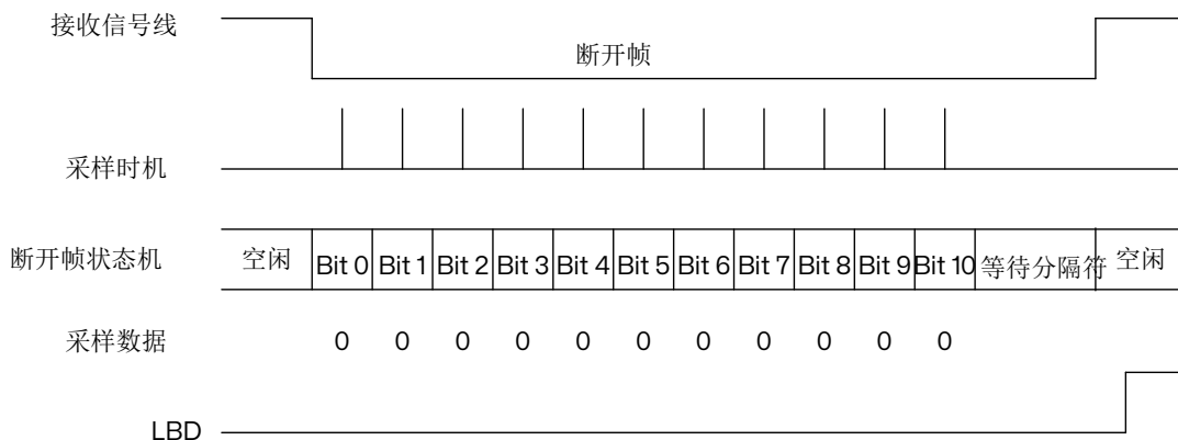
图 25.7 说明了断开符号检测器状态机的行为和断开符号标志的关系。
