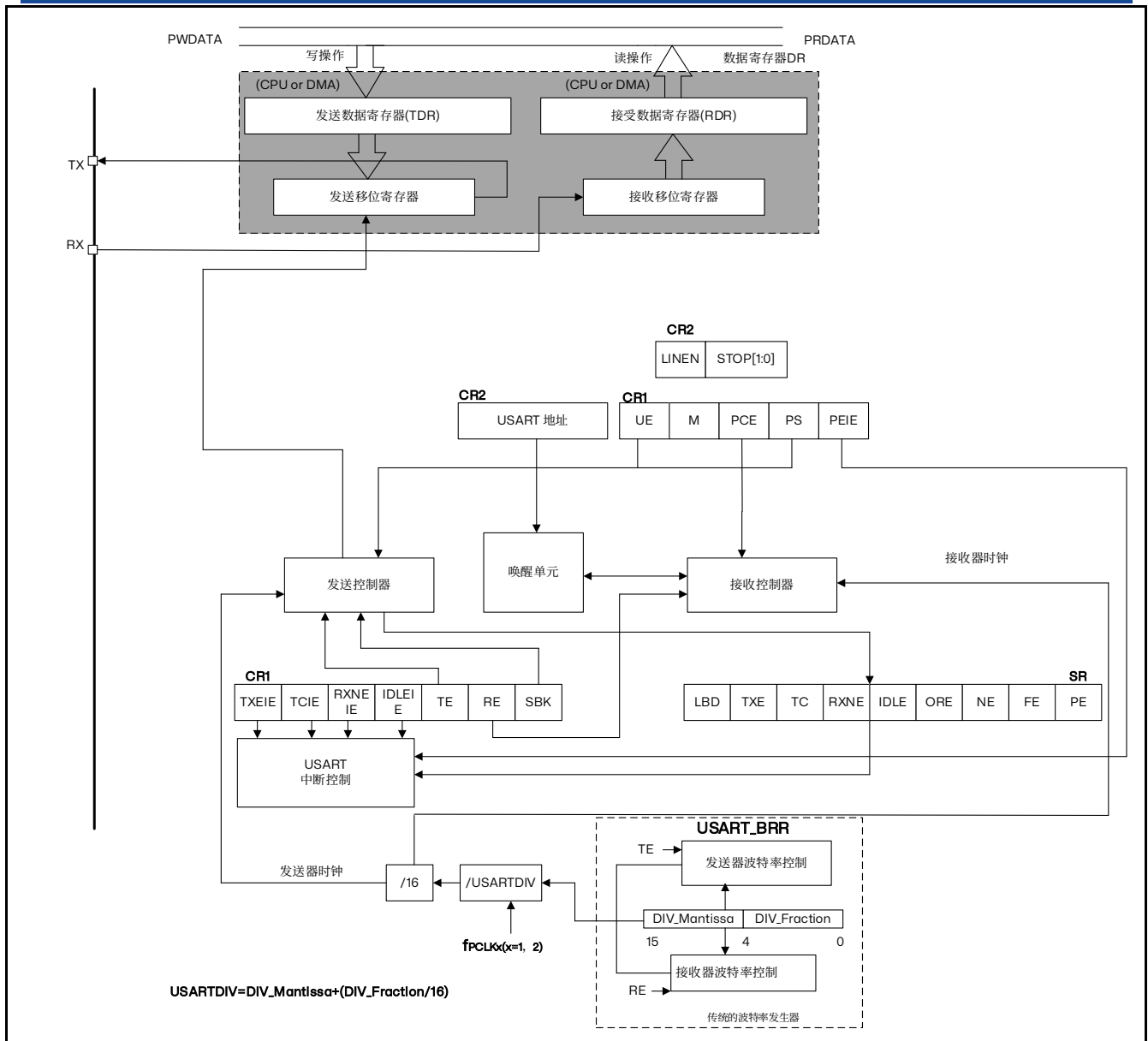
图 25.1 UART 框图
