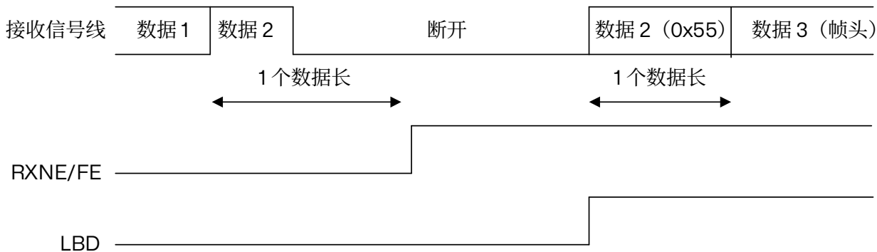
图 25.8 给出了一个断开帧的例子。
