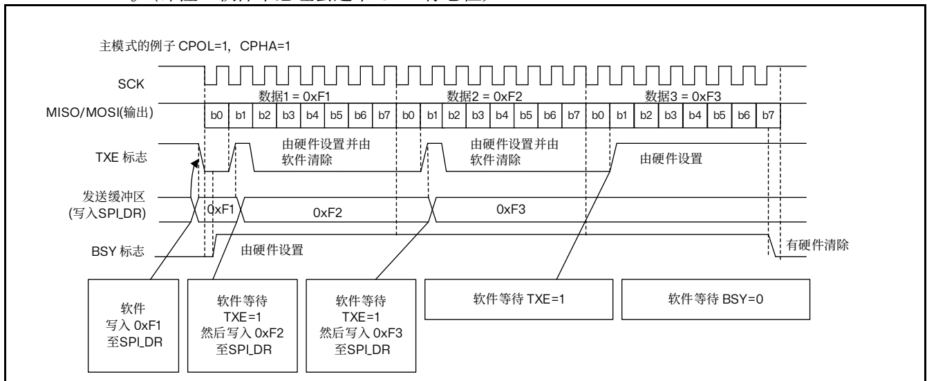
图 23.7 主设备只发送模式 (BIDIMODE=0 并且 RXONLY=0) 下连续传输时，TXE/BSY 变化示意图
