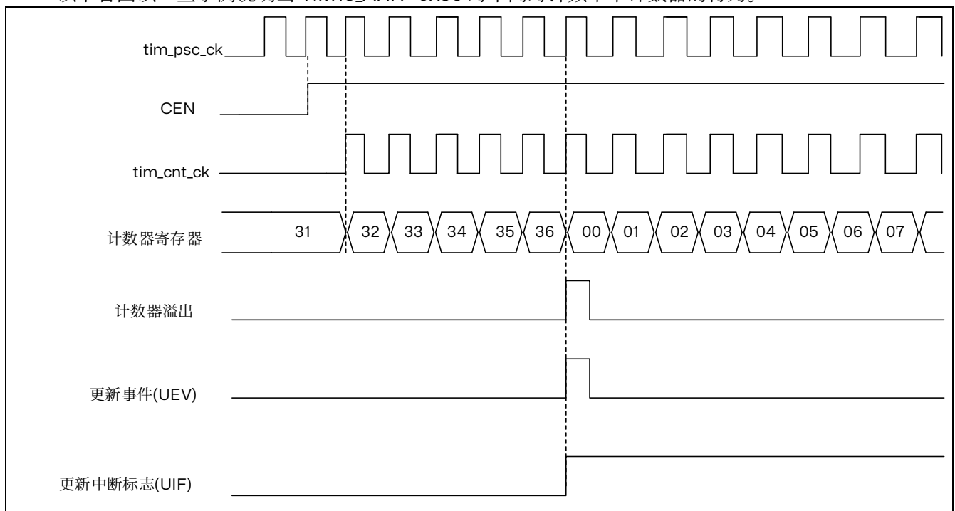
图 16.4 计数器时序图，内部时钟分频因子为 1
