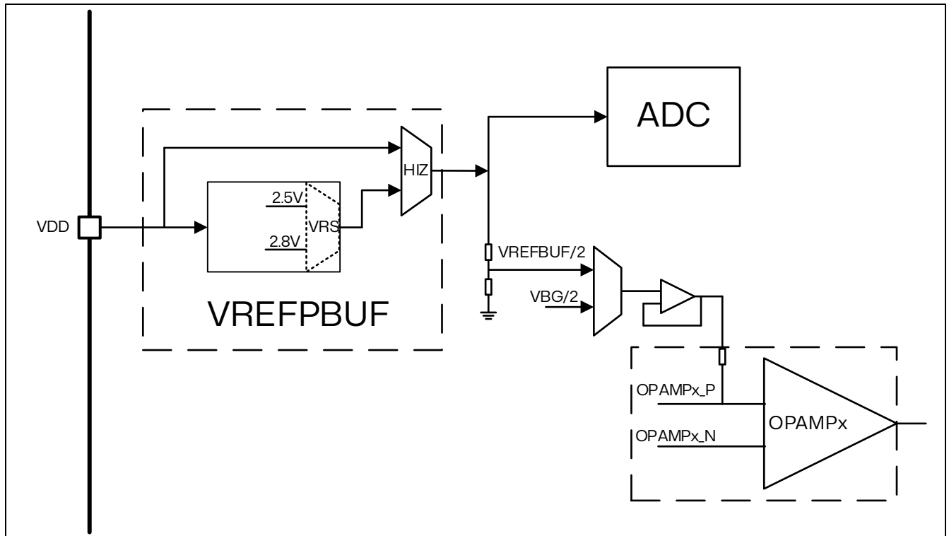
图 12.1 VREFBUF 框图
