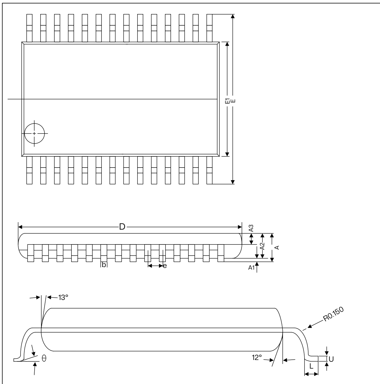
图 6.1 轮廓图
