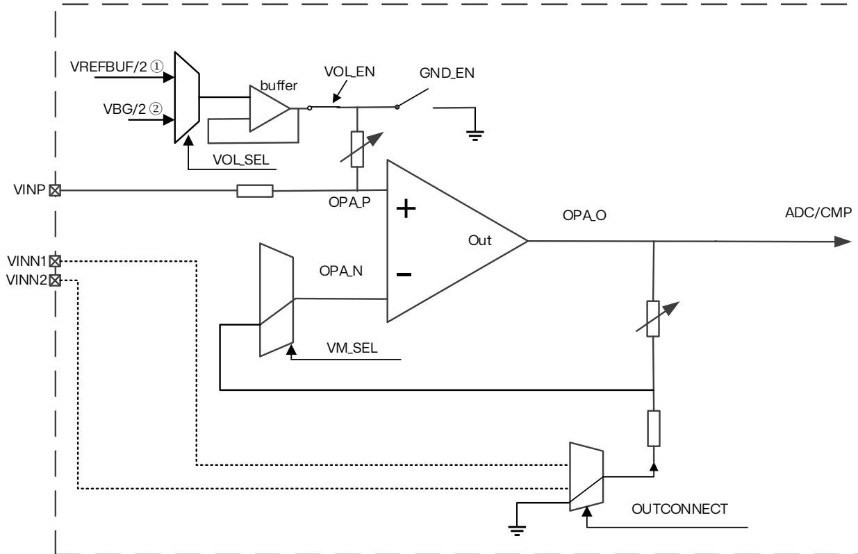
图 18.8 OPAMP1/OPAMP2 PGA 模式 (P-偏置, N-GND)
