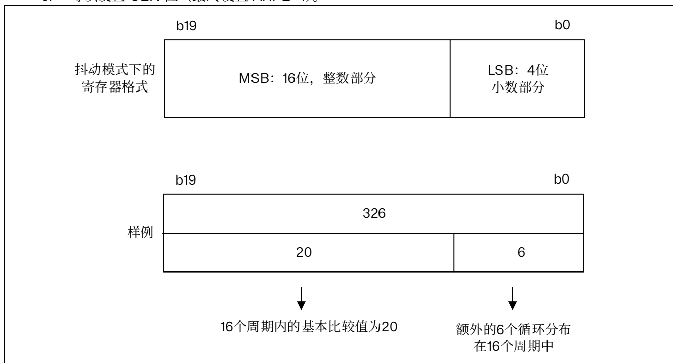
图 14.33 抖抖模式下的数据格式和寄存器编码
