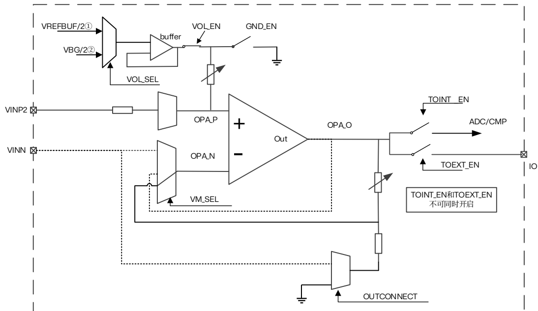
图 18.9 OPAMP3 PGA 模式 (P-偏置, N-GND)
