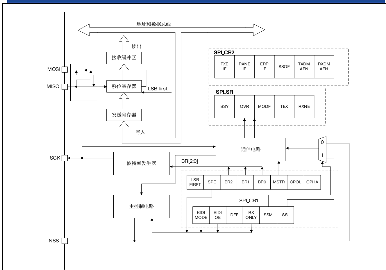
图 23.1 SPI 框图
