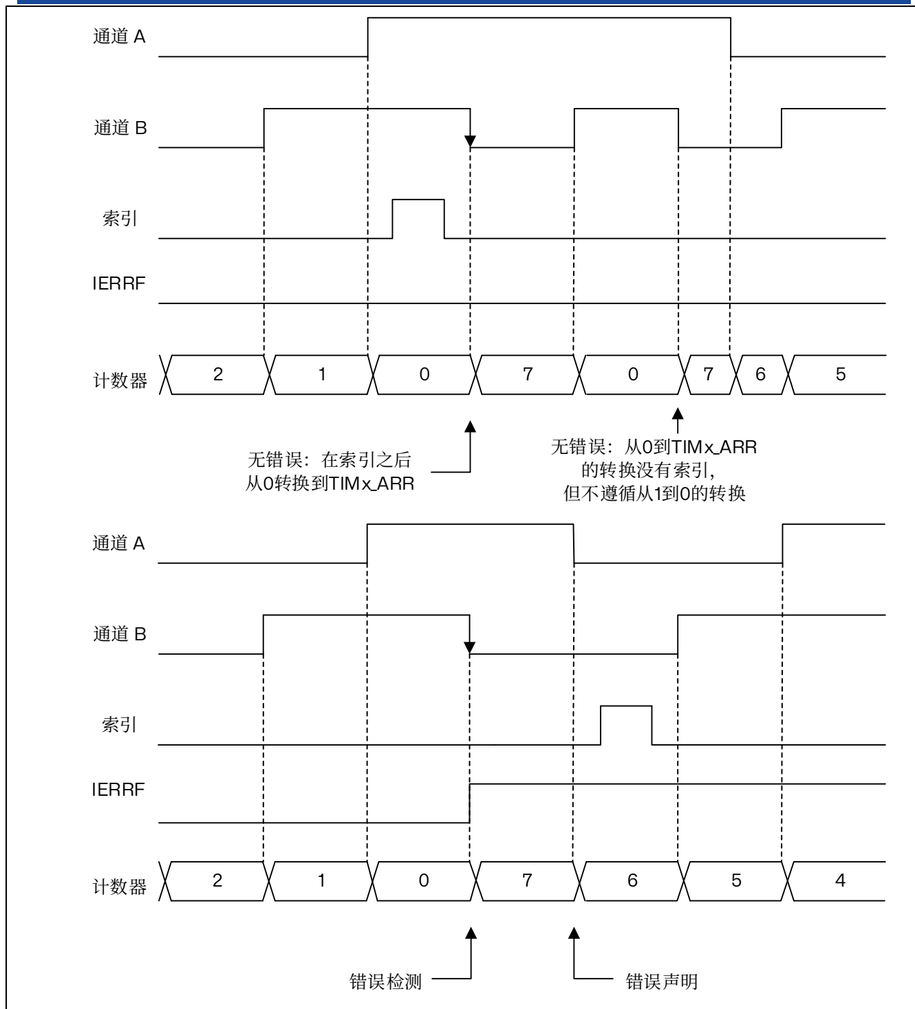
图 15.73 递减计数编码器错误检测
