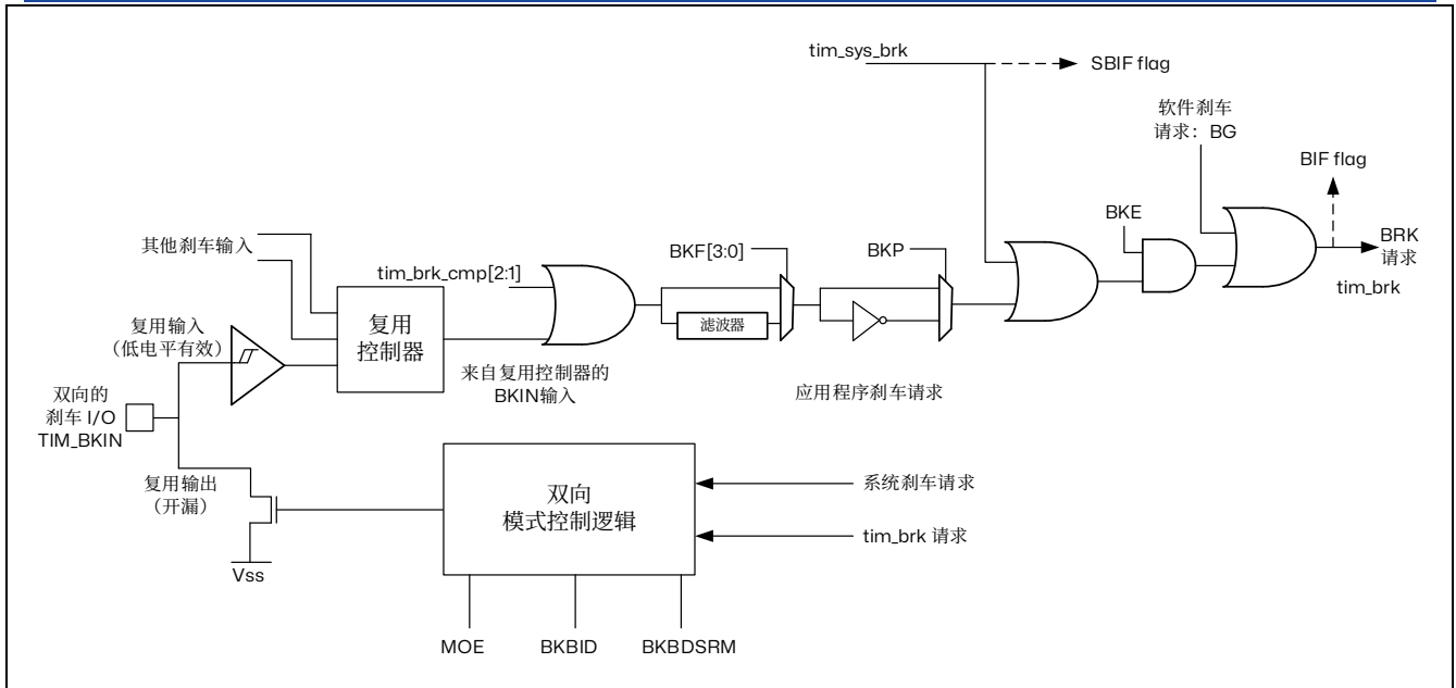
图 16.32 输出重定向
