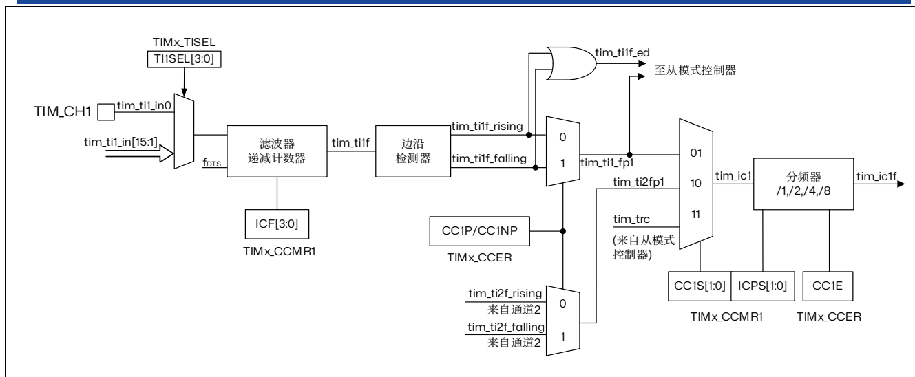
图 15.27 捕获/比较通道（如：通道 1 输入部分）
