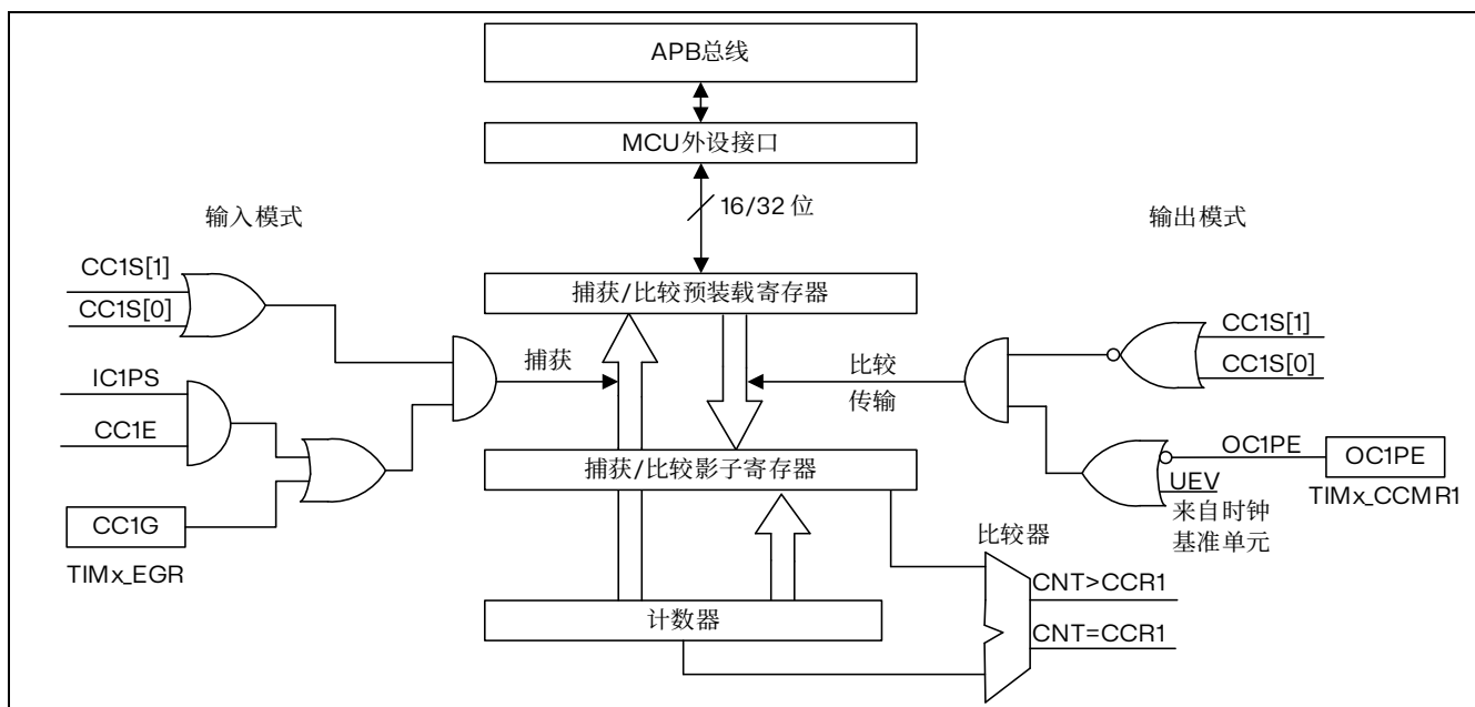
图 15.28 捕获/比较通道 1 的主电路
